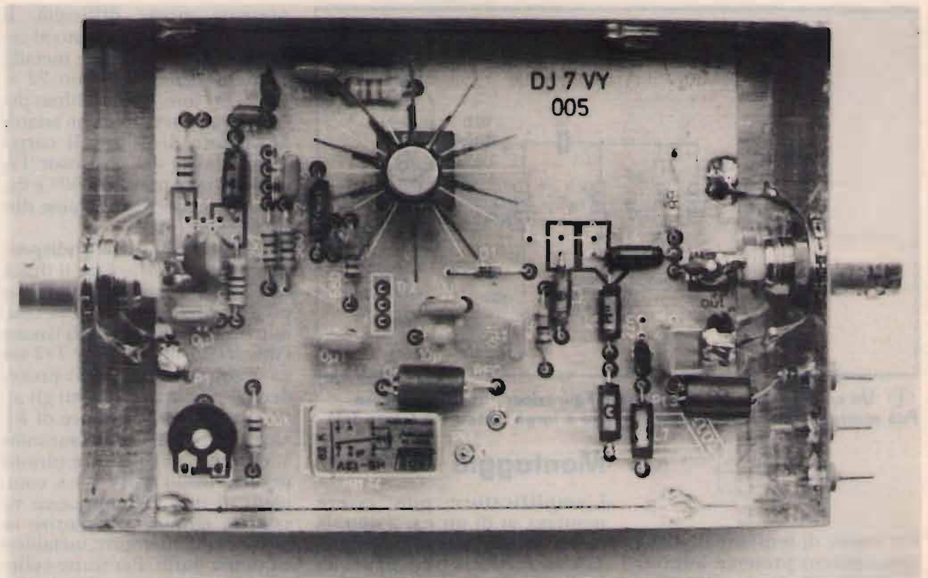
⑦ Aspetto dell'amplificatore a montaggio ultimato.
