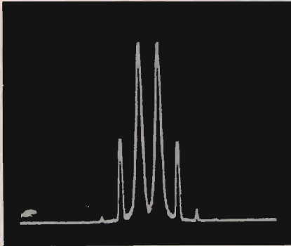
② Reiezione-IM a pieno pilotaggio misurata a 3,6 MHz con U_D = 30 V; orizzontale: 20 kHz/div. - verticale: 10 dB/div.
