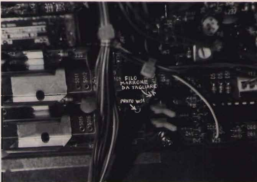
① Circuiteria presente nella parte inferiore dell'IC765 (zona nei pressi dei filtri e sedi filtri FL 102/101 opzionali - punto W 31)
