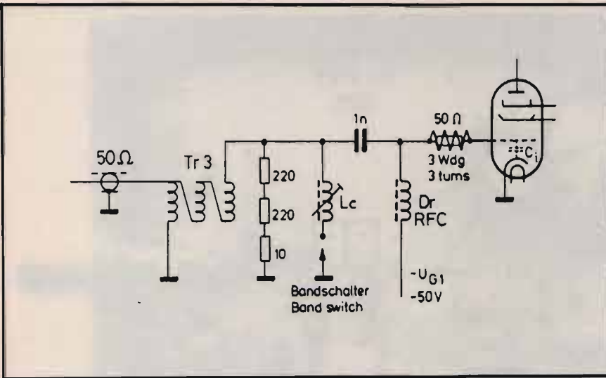
⑤ Un amplificatore a valvola in configurazione. Catodo a massa. Può essere pilotato con un trasformatore a larga banda Tr3 (come Tr1).
